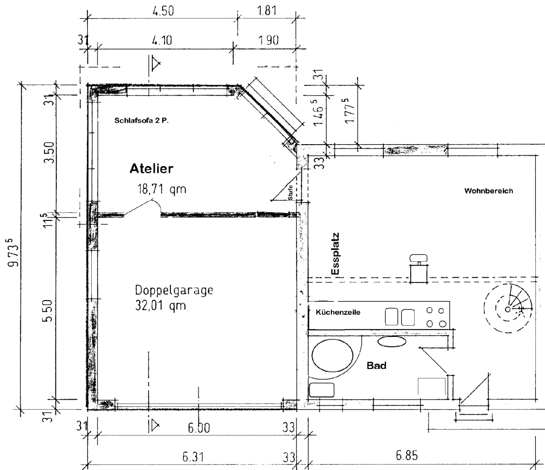
Grundriss
